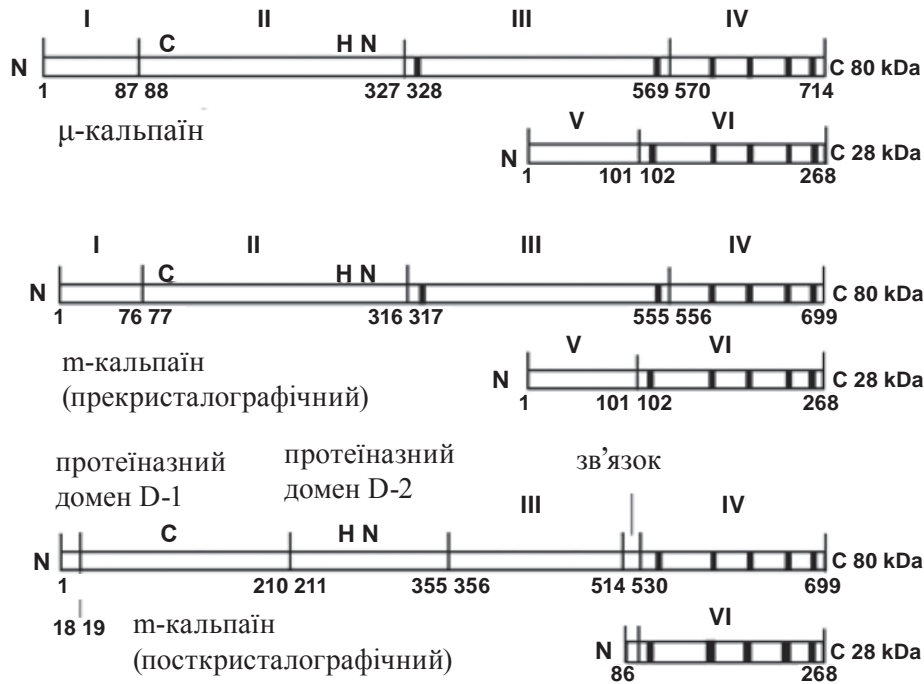
Схема доменної будови типових кальпаїнів людини [2, 9]
